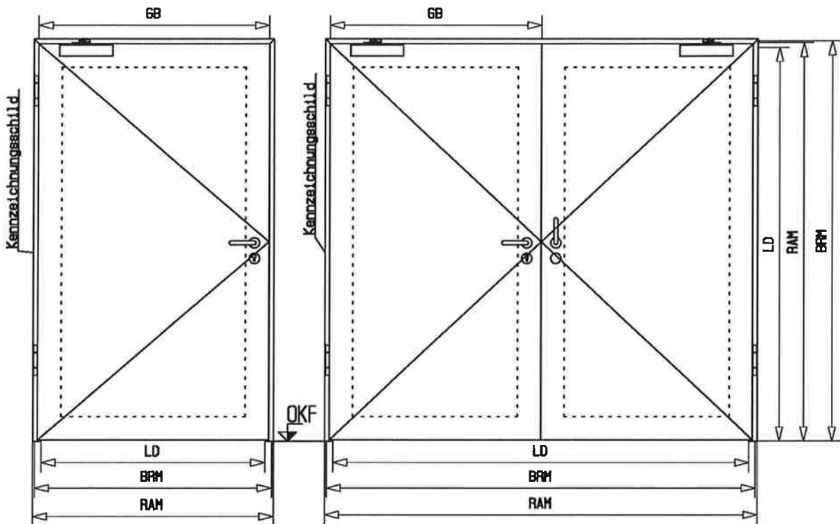
dargestellt: Gangflügel DIN links Gangflügel DIN rechts im Spiegelbild
